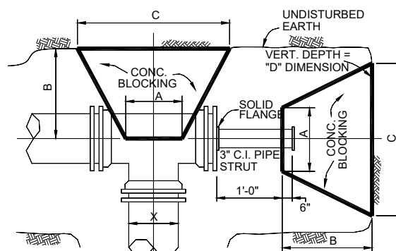
TEES
